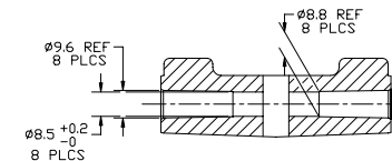
SECTION D-D
